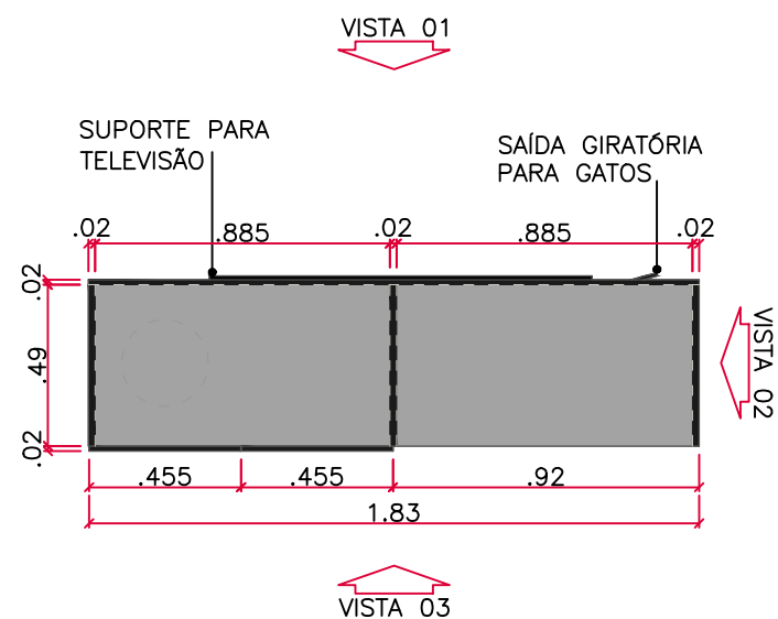
MA-08 PLANTA BAIXA
