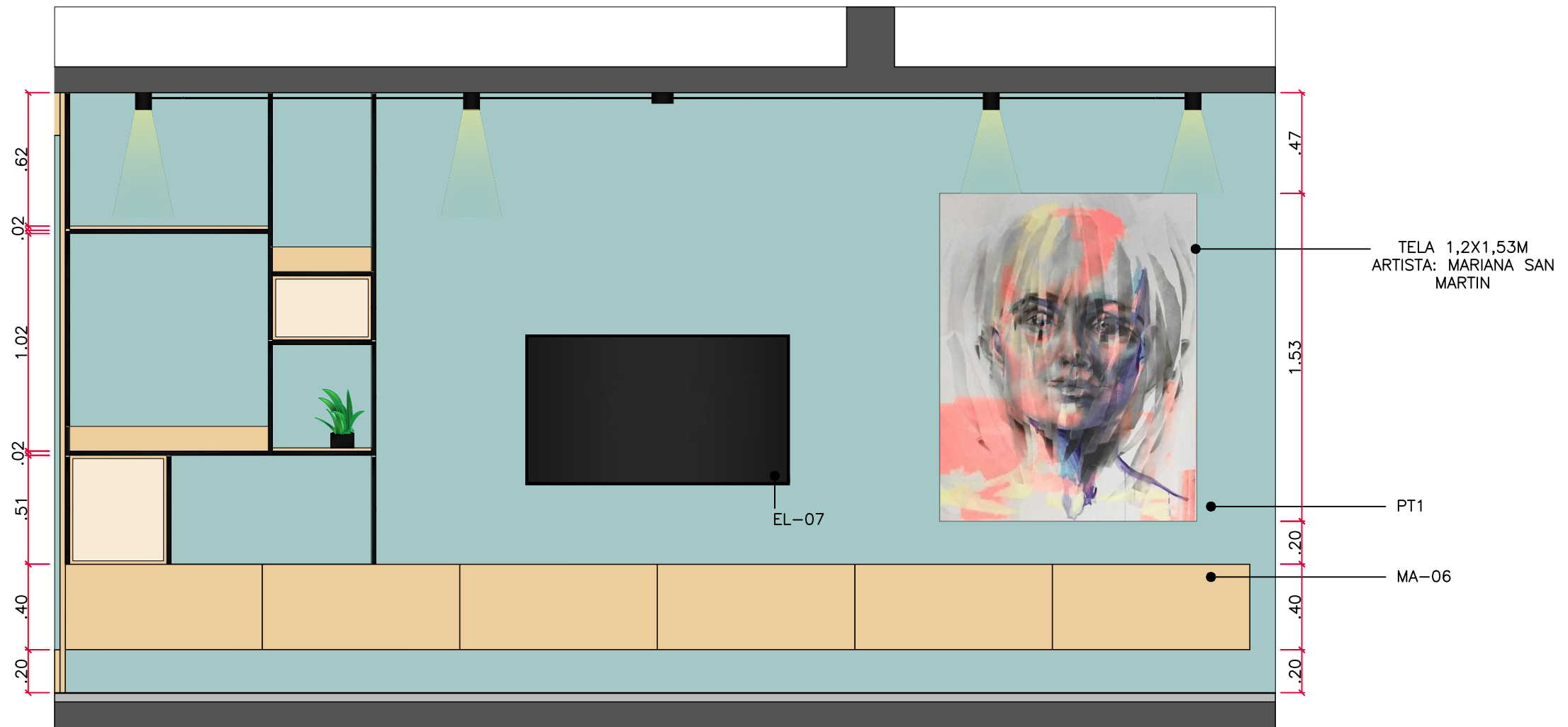
VISTA 01 - SALA DE ESTAR / JANTAR esc 1:25
