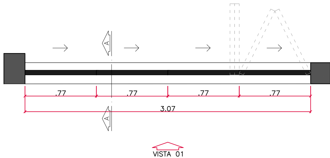
J1 - PLANTA BAIXA
