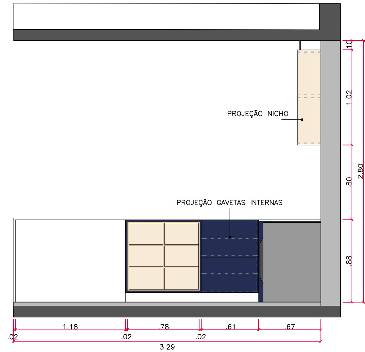
MA-02 E 03 VISTA 02 esc 1:25
