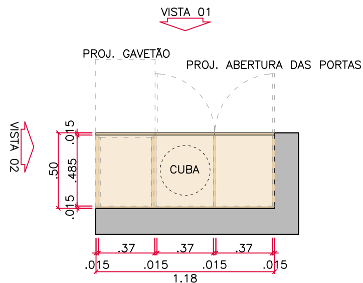
MA-13 PLANTA BAIXA esc 1:25
