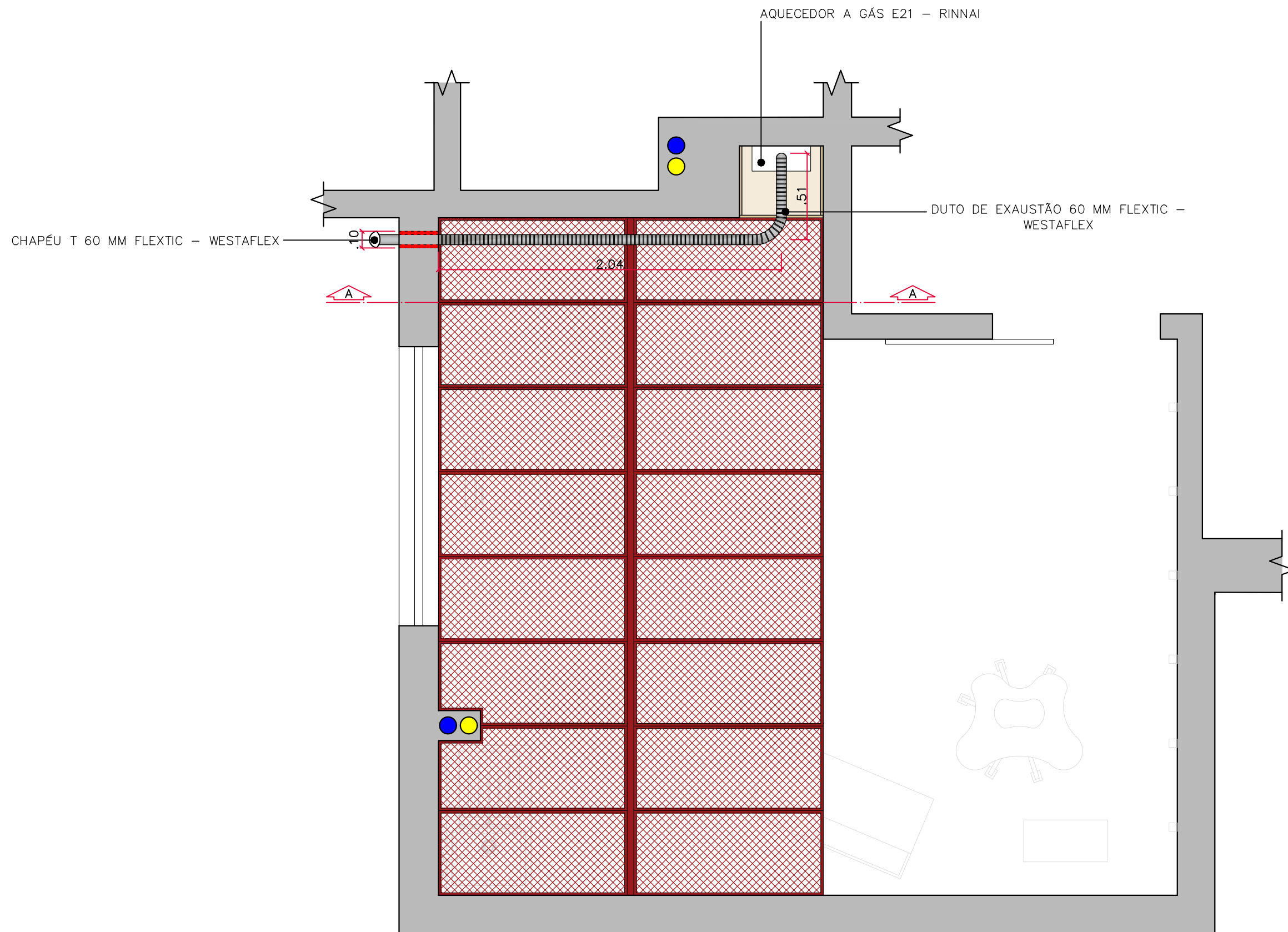
PLANTA BAIXA - INSTALAÇÃO DO AQUECEDOR A GÁS esc 1:25
