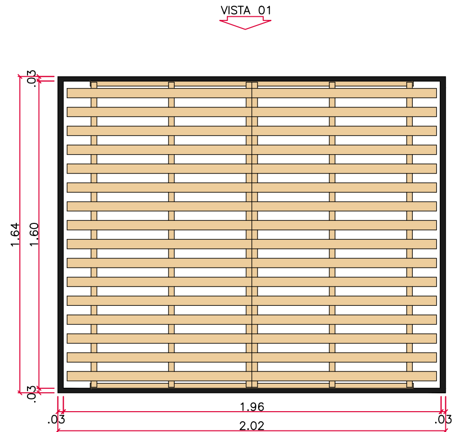
MA-10 PLANTA BAIXA esc 1:20
