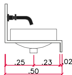
BN - 04 VISTA 02 esc 1:20
