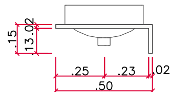
BN - 03 VISTA 02 esc 1:20
