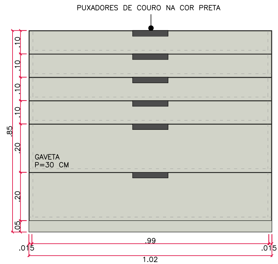
MA-12 VISTA 01 esc 1:10
