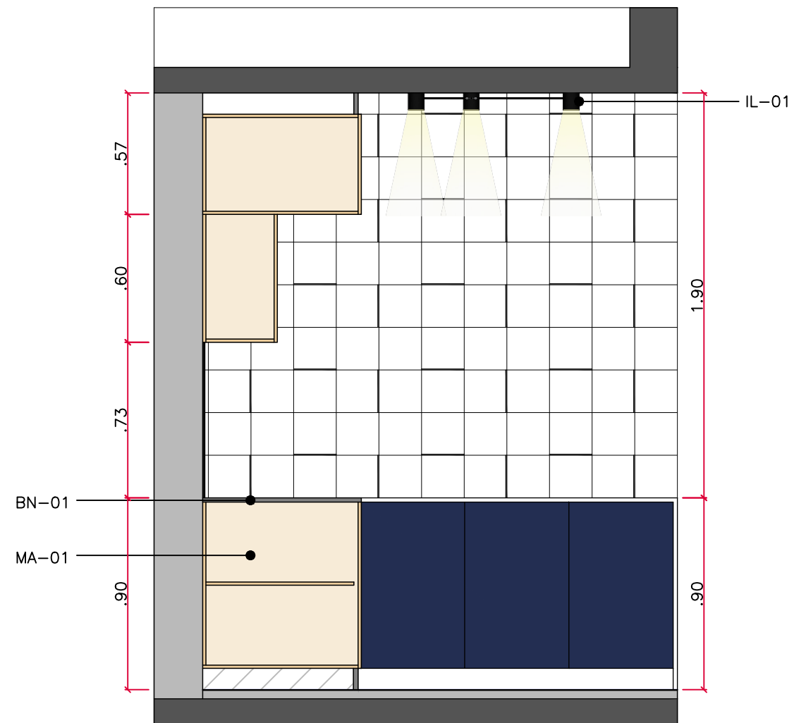
VISTA 04 - SERVIÇO esc 1:25
