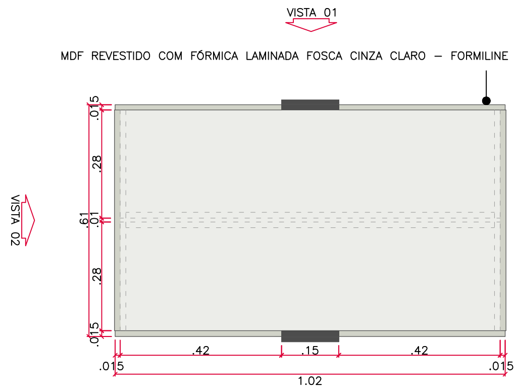
MA-12 PLANTA BAIXA esc 1:10
