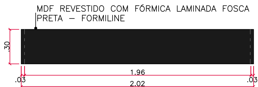
MA-10 VISTA 01 esc 1:20
