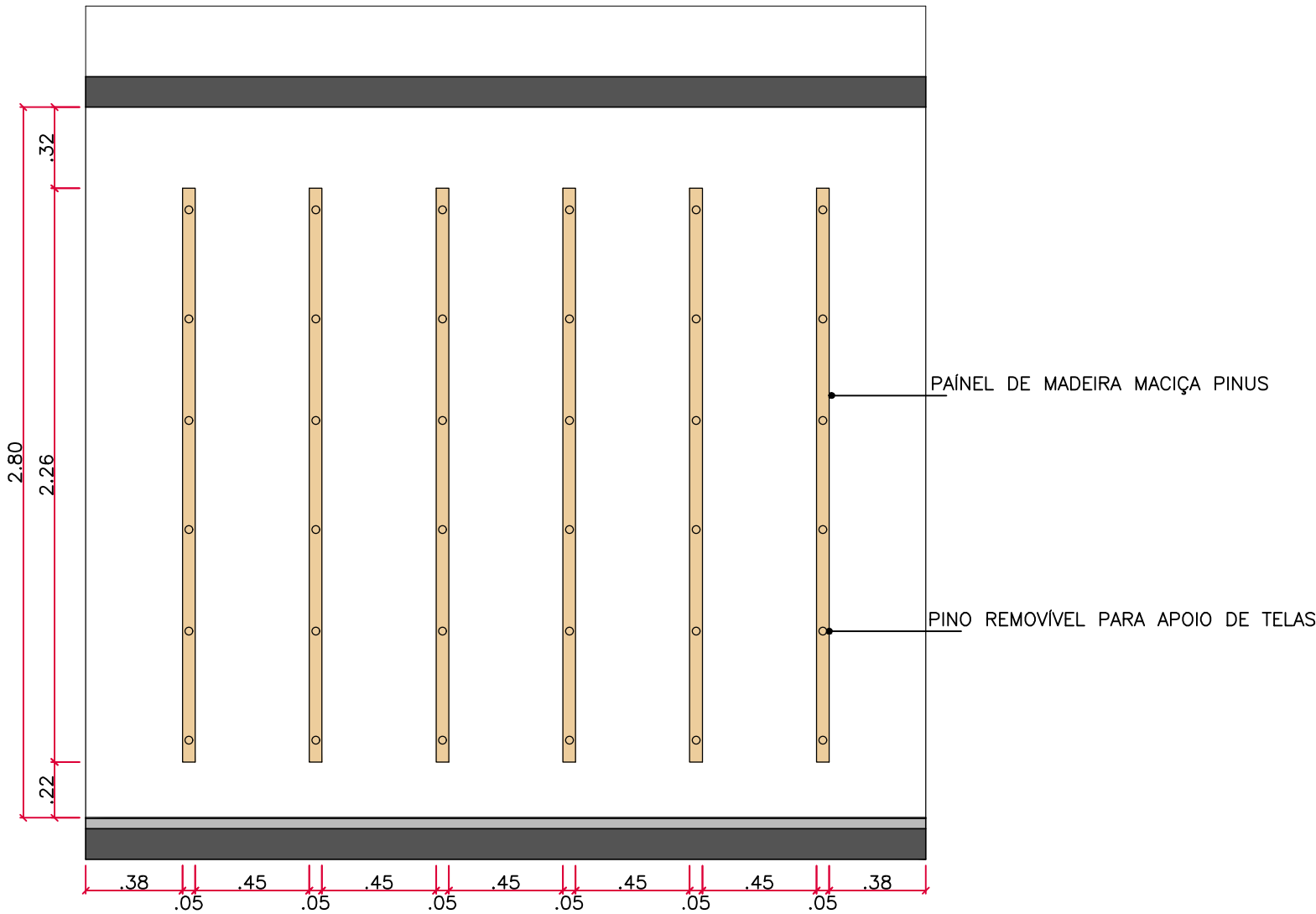
MA-18 VISTA 01 esc 1:25
