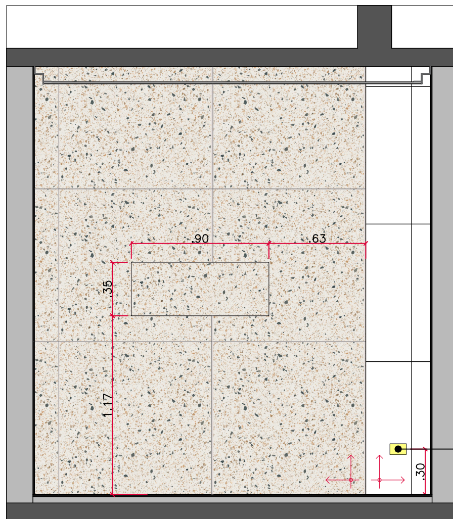
VISTA 02 - BANHEIRO esc 1:25
