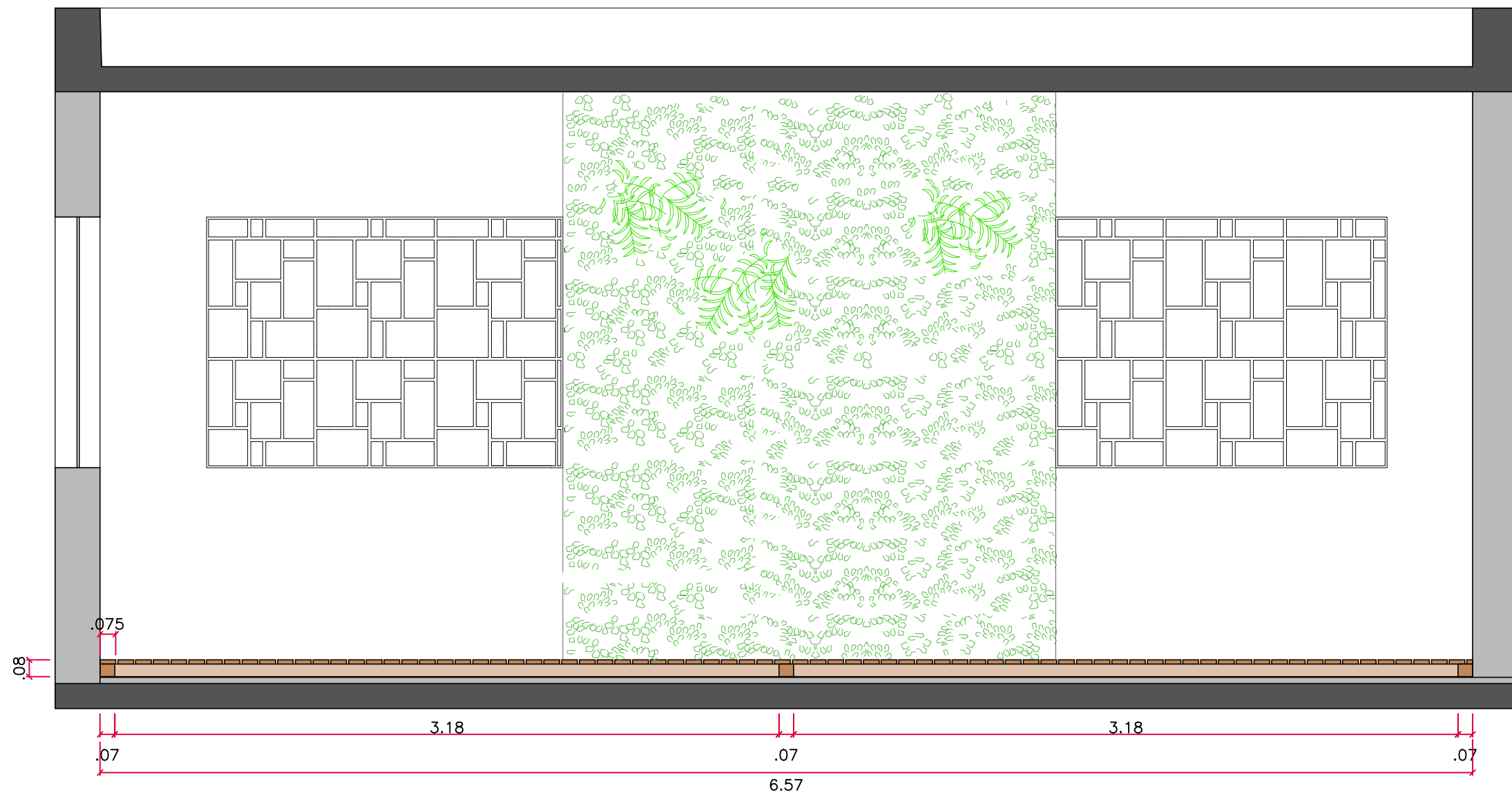
CORTE BB - DECK esc 1:25
