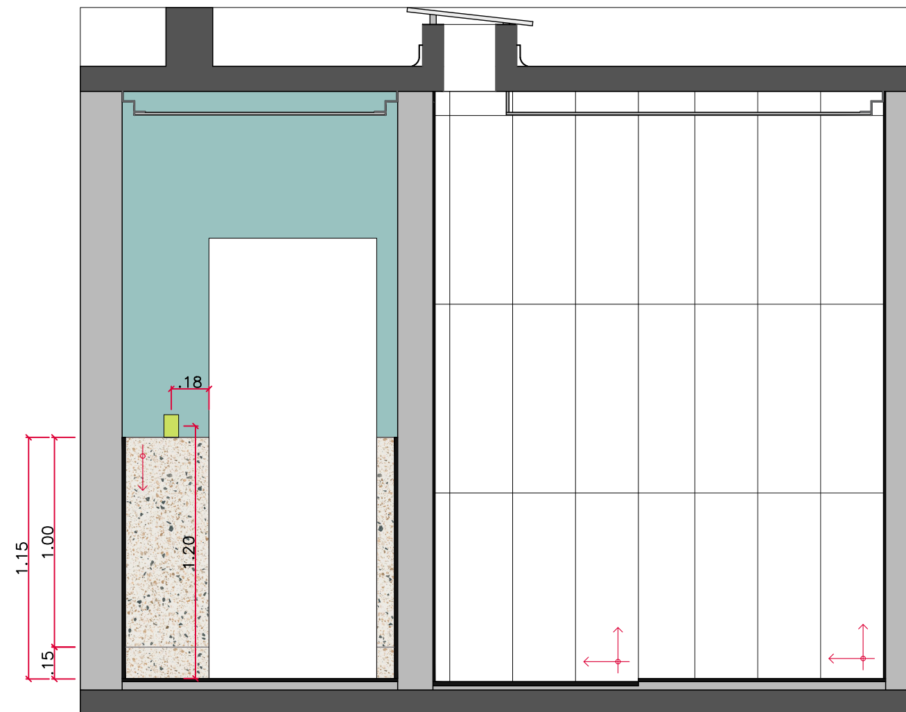
VISTA 03 - BANHEIRO esc 1:25
