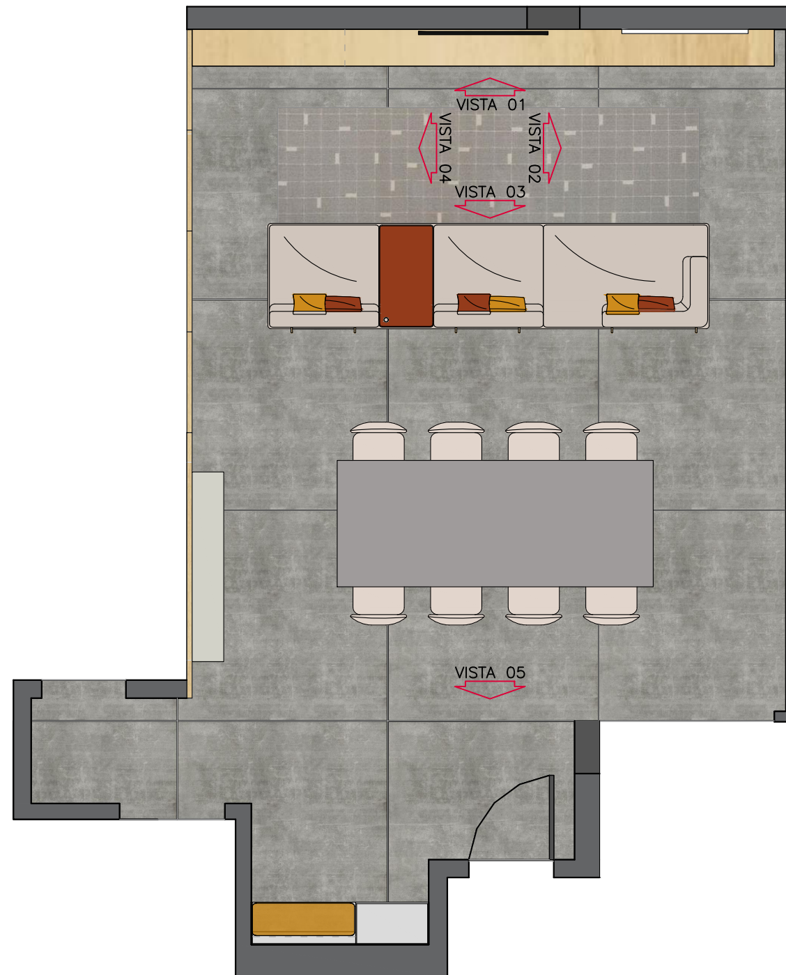
PLANTA BAIXA - SALA DE ESTAR / JANTAR esc 1:50
