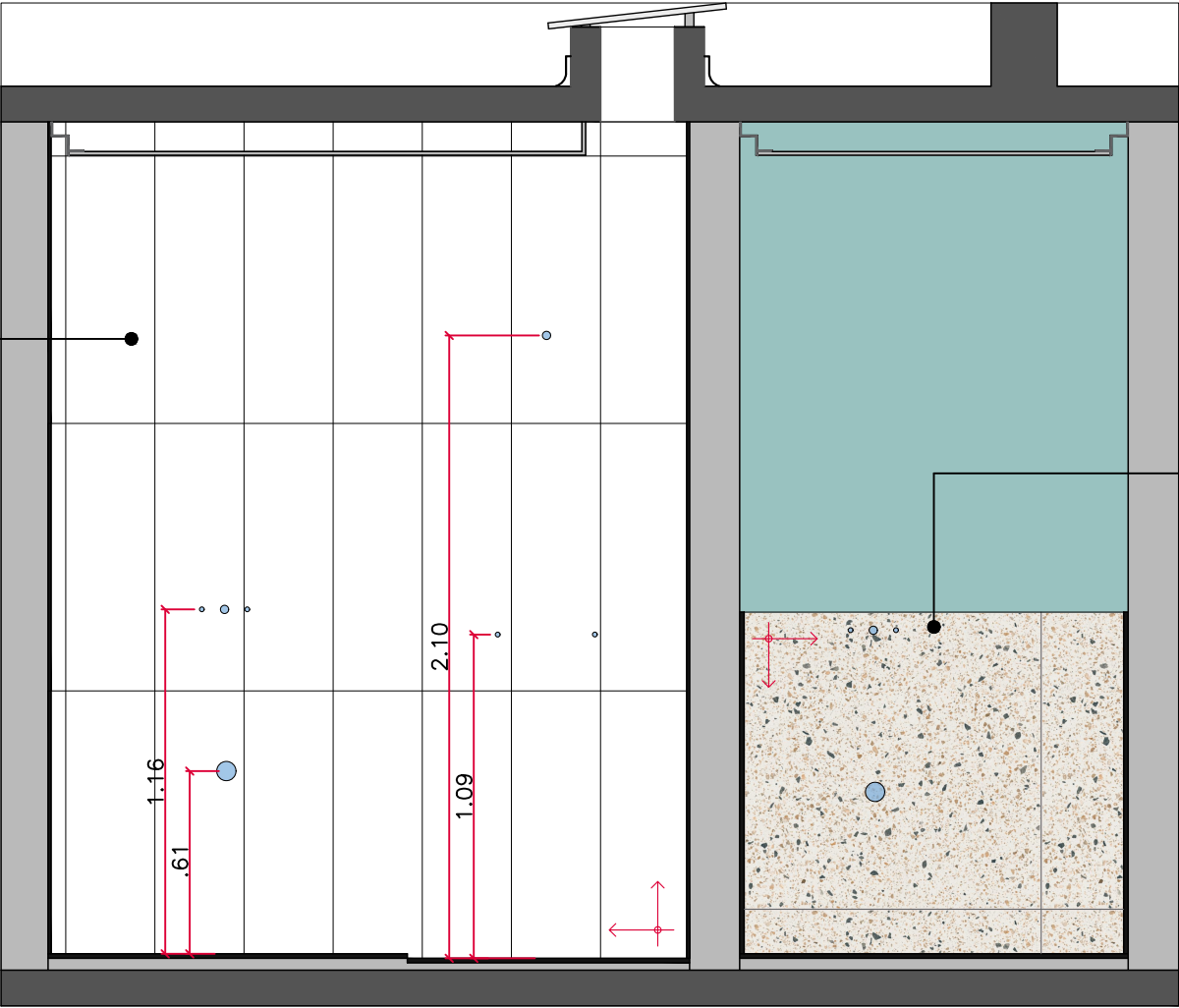
VISTA 01 - BANHEIRO esc 1:25
