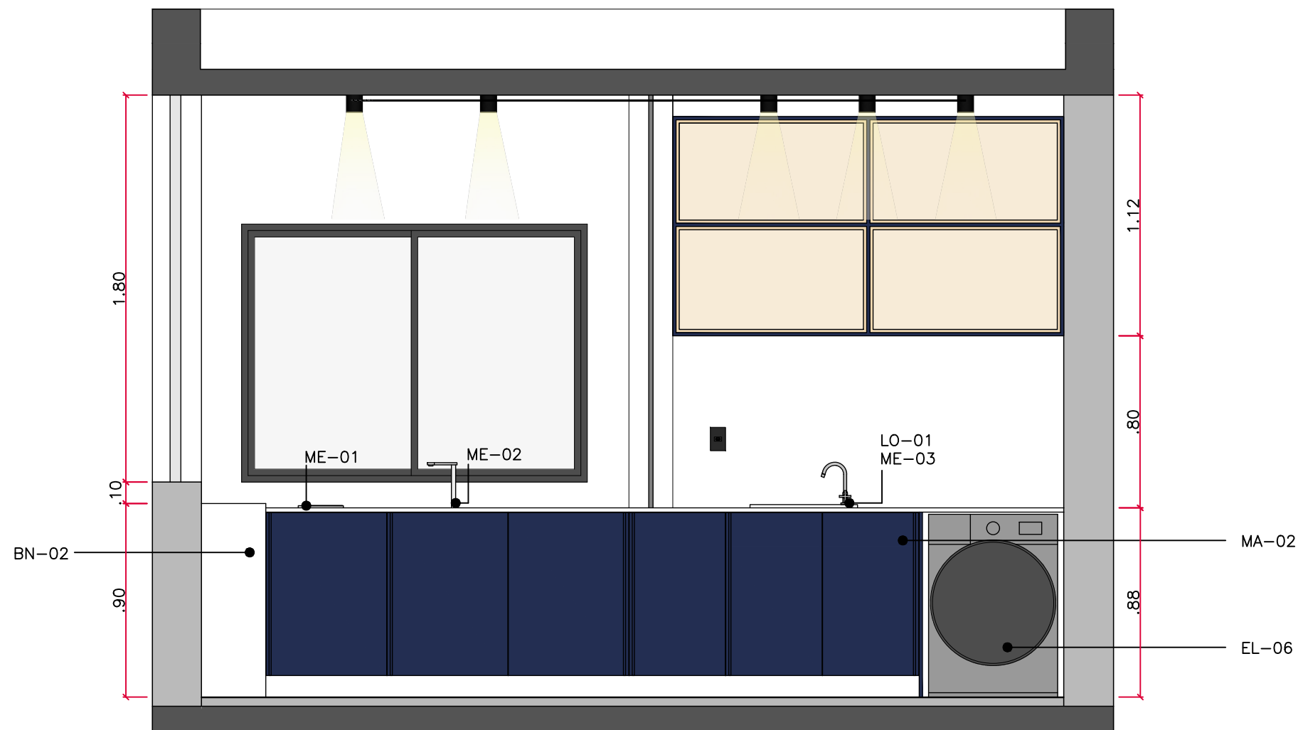
VISTA 02 - SERVIÇO esc 1:25
