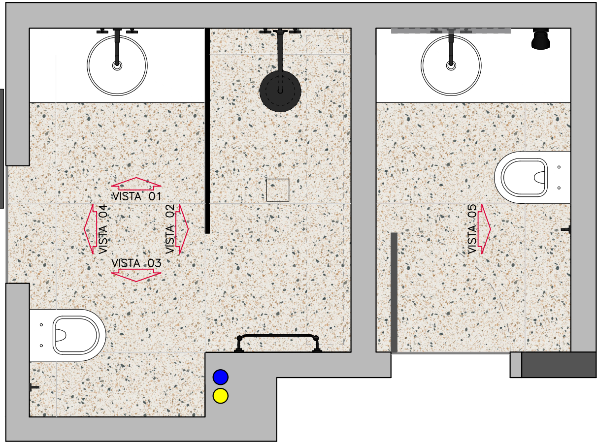
PLANTA BAIXA - BANHEIRO esc 1:25
