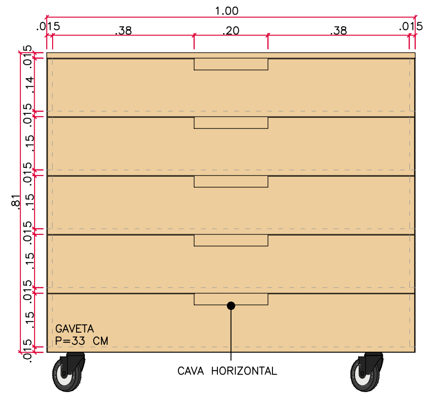
MA-16 VISTA 01 esc 1:10
