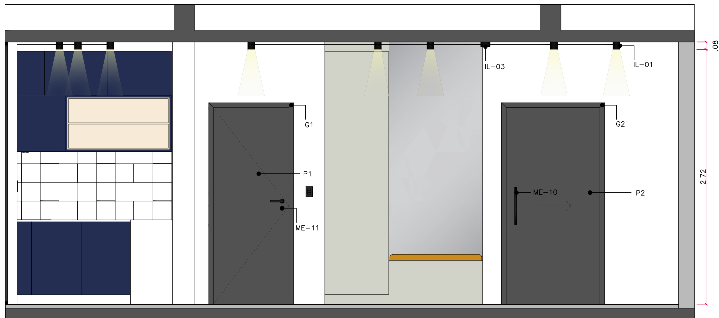
VISTA 04 - SALA DE ESTAR / JANTAR esc 1:25
