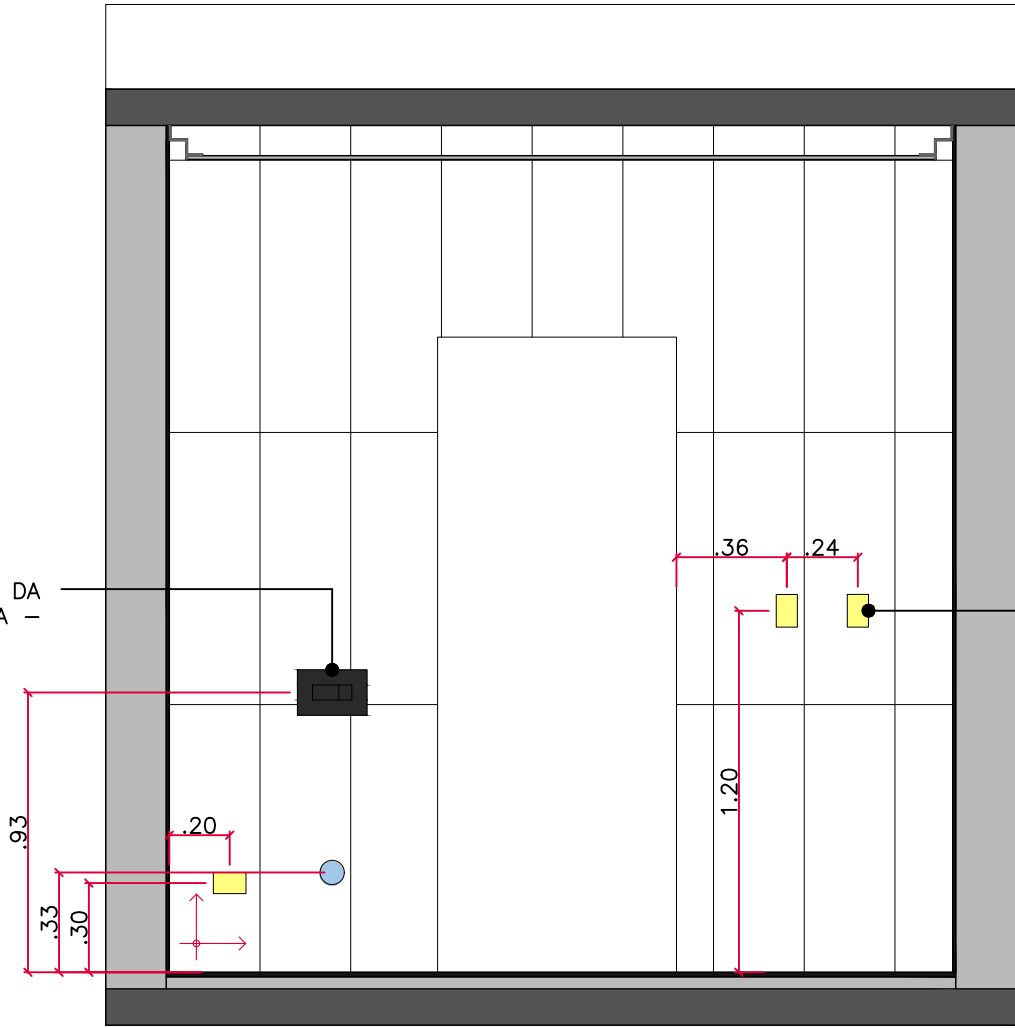
VISTA 04 - BANHEIRO esc 1:25
