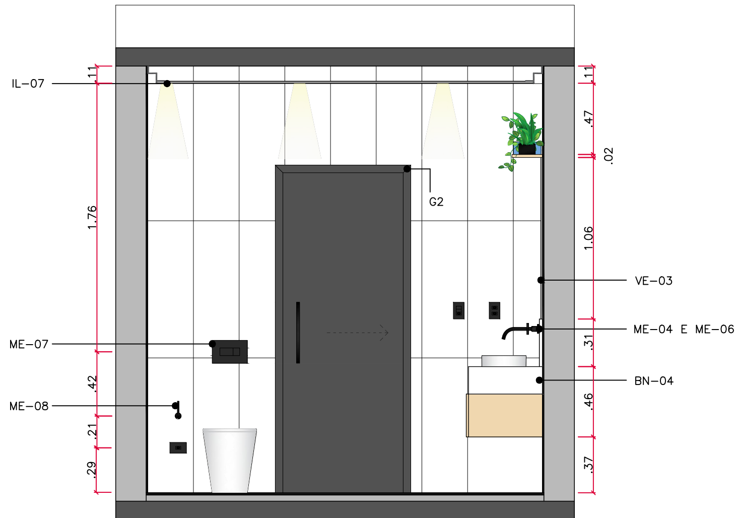
VISTA 04 - BANHEIRO esc 1:25
