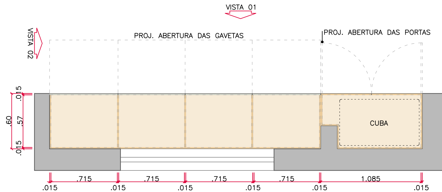
MA- 15 PLANTA BAIXA
