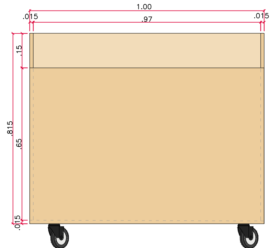
MA-16 VISTA 03 esc 1:10
