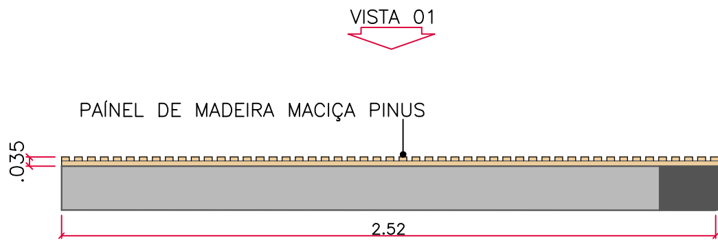
MA-06 PLANTA BAIXA esc 1:20
