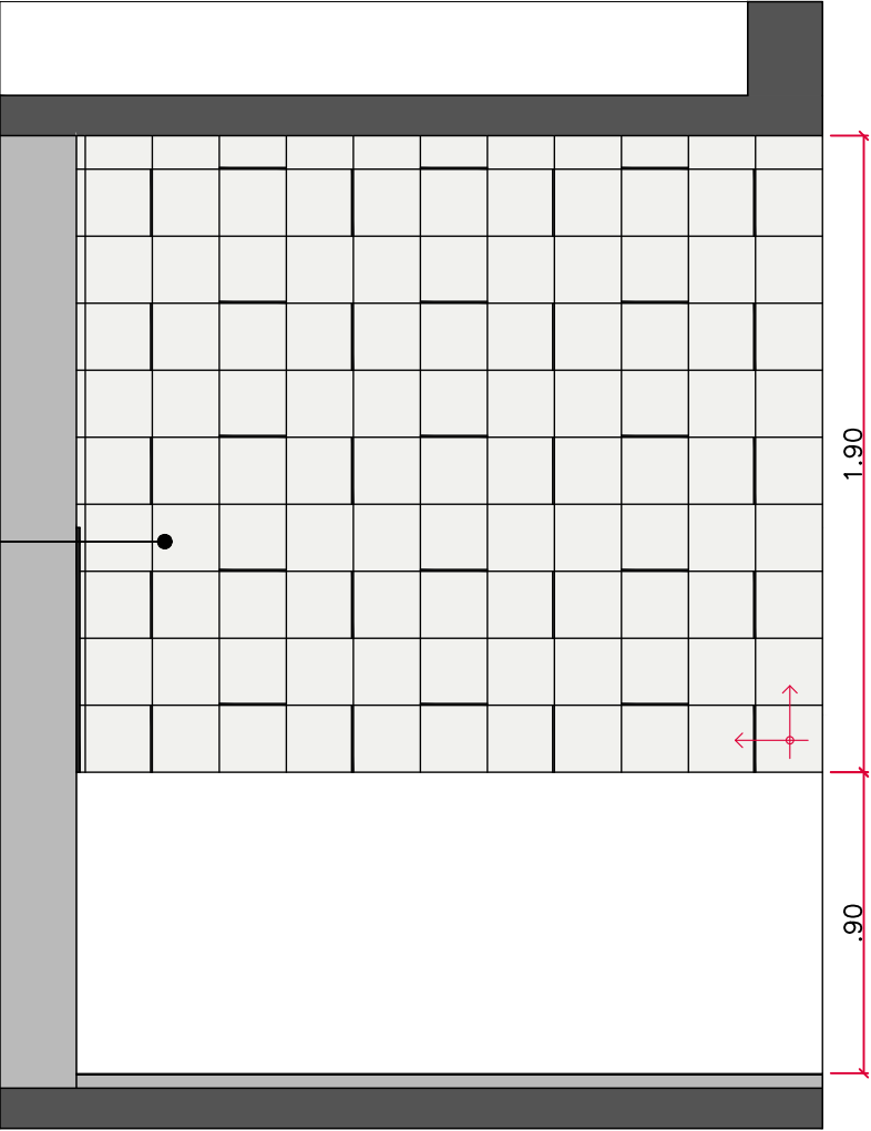
VISTA 03 - SERVIÇO esc 1:25
