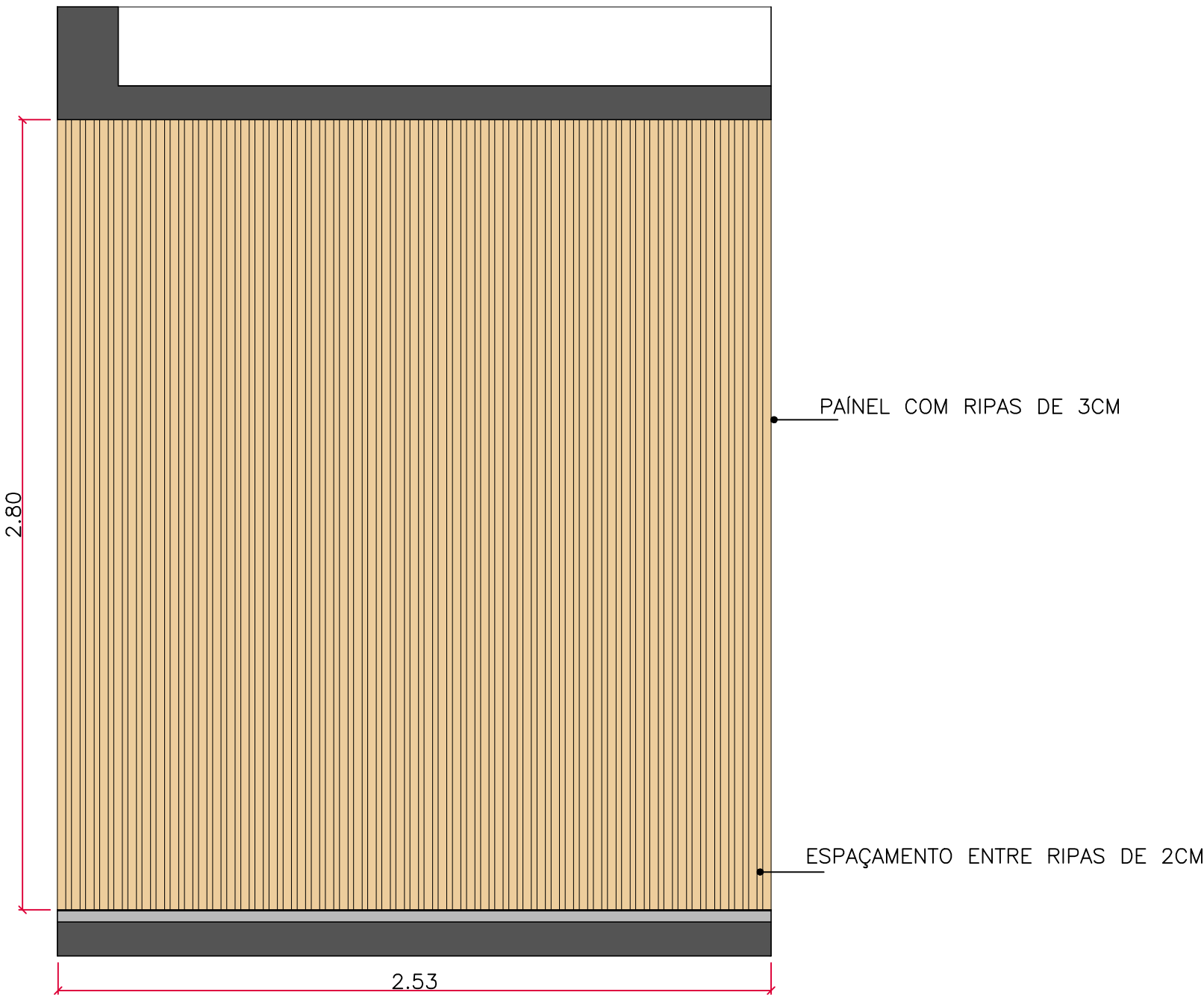
MA-06 VISTA 01 esc 1:25
