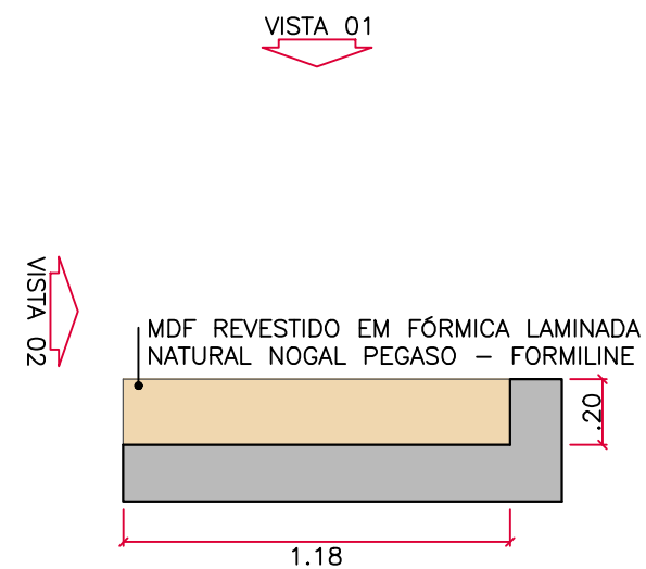
MA-14 PLANTA BAIXA esc 1:25
