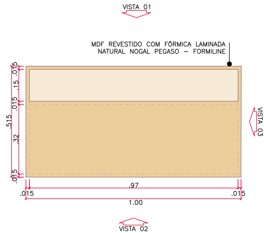
MA-16 PLANTA BAIXA esc 1:10
