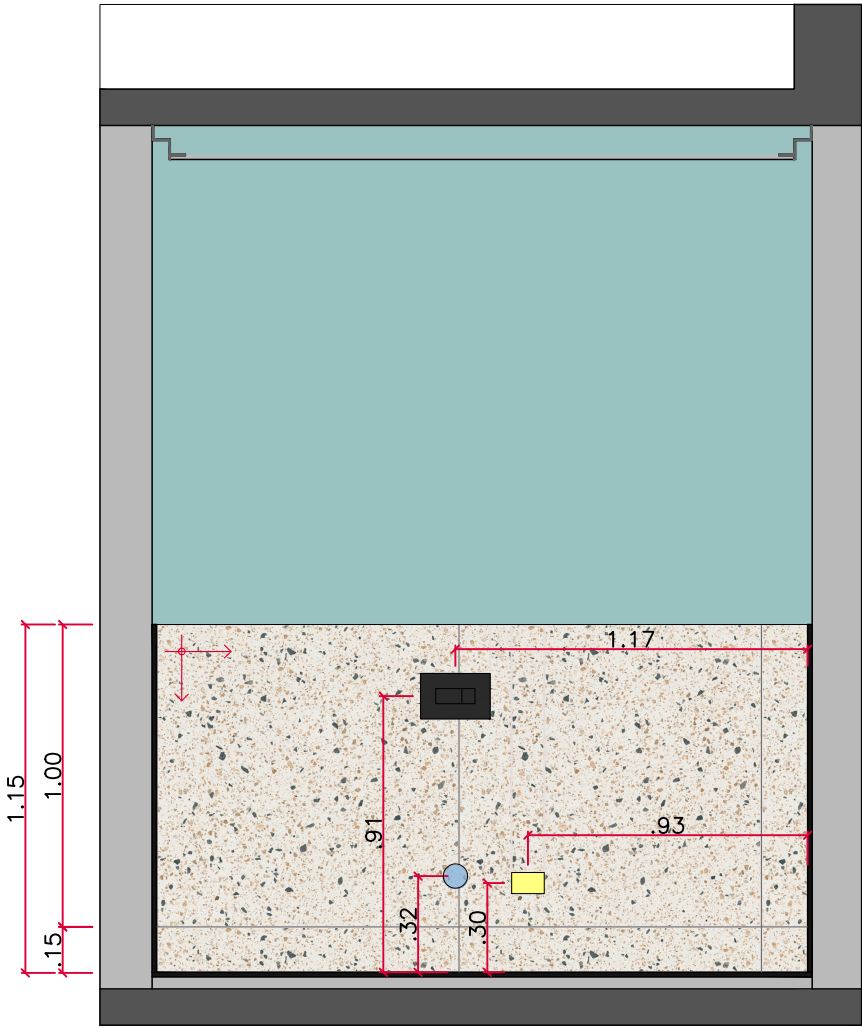
VISTA 05 - BANHEIRO esc 1:25
