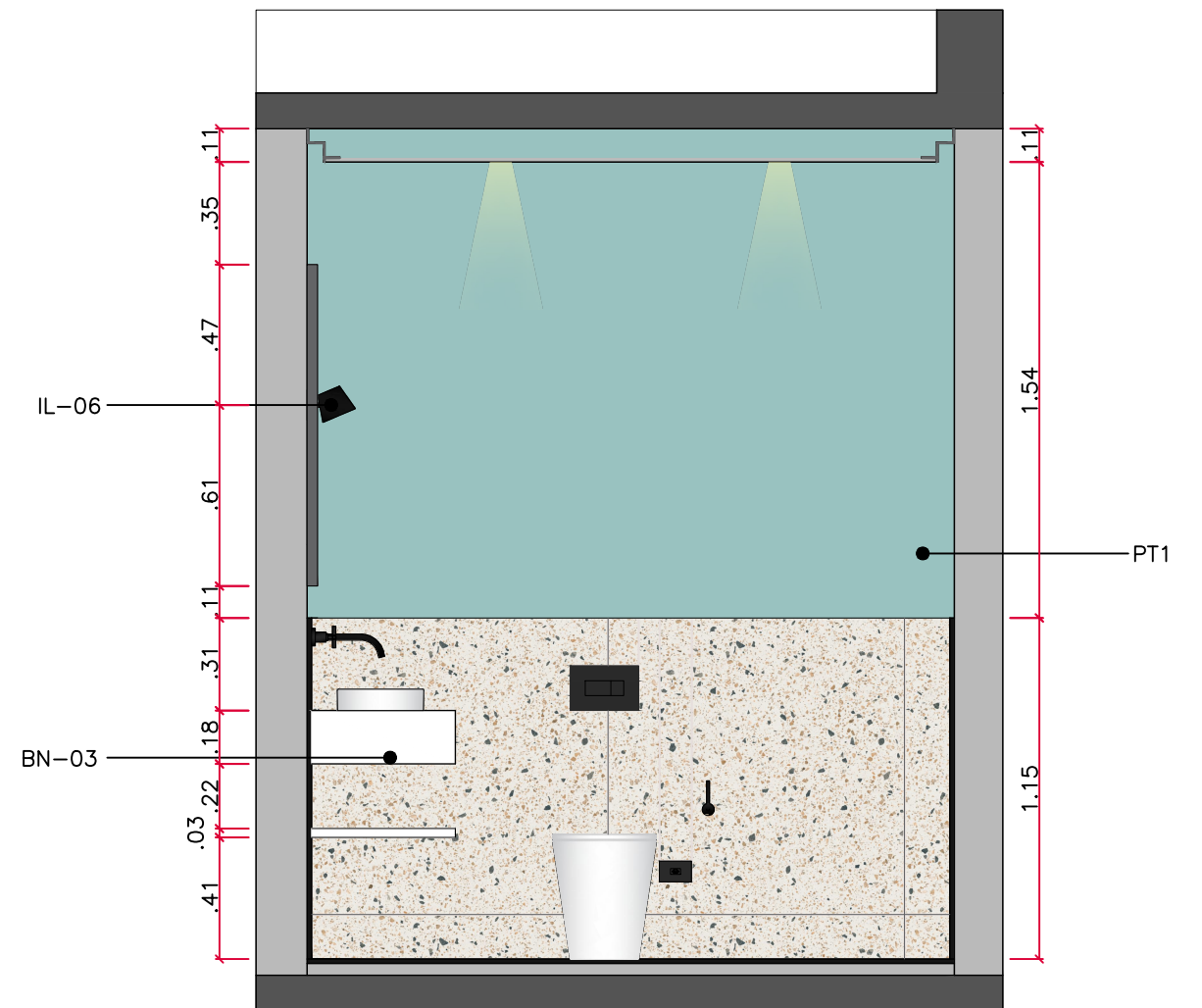
VISTA 05 - BANHEIRO esc 1:25
