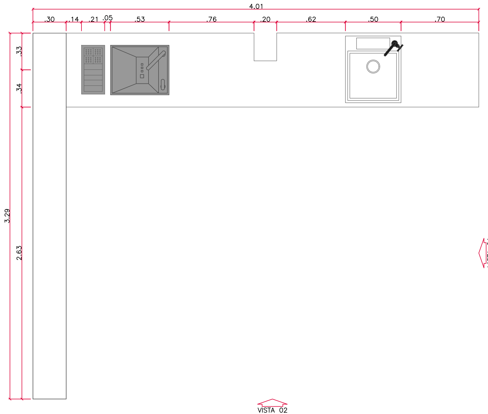
BN - 02 PLANTA BAIXA esc 1:20
