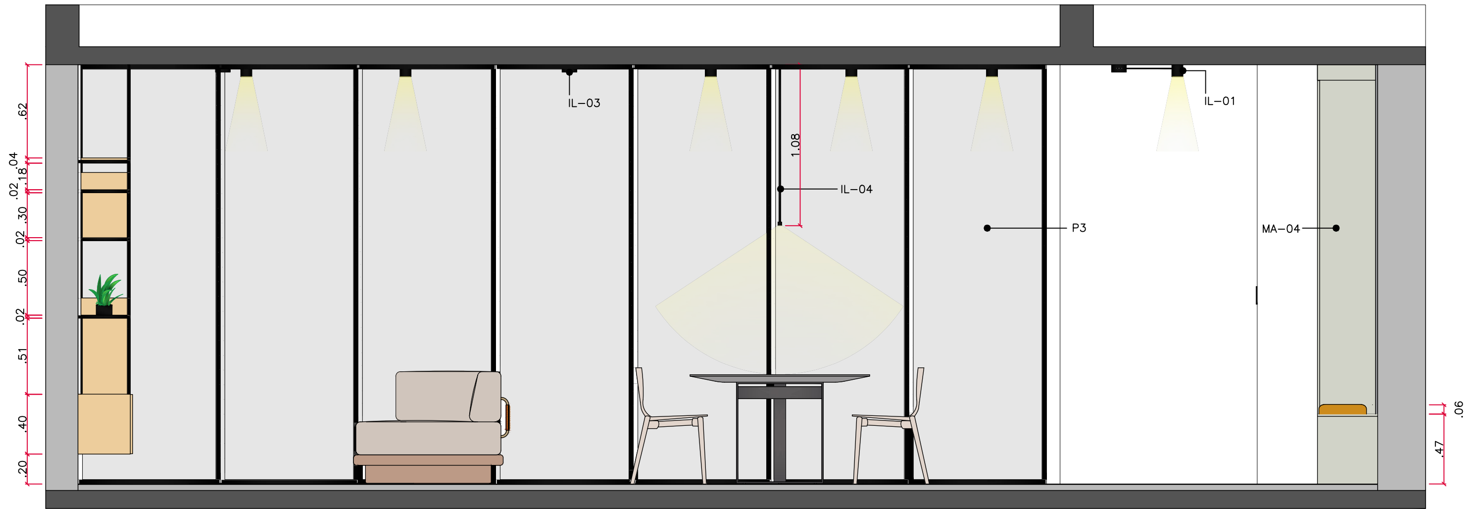
VISTA 02 - SALA DE ESTAR / JANTAR esc 1:25
