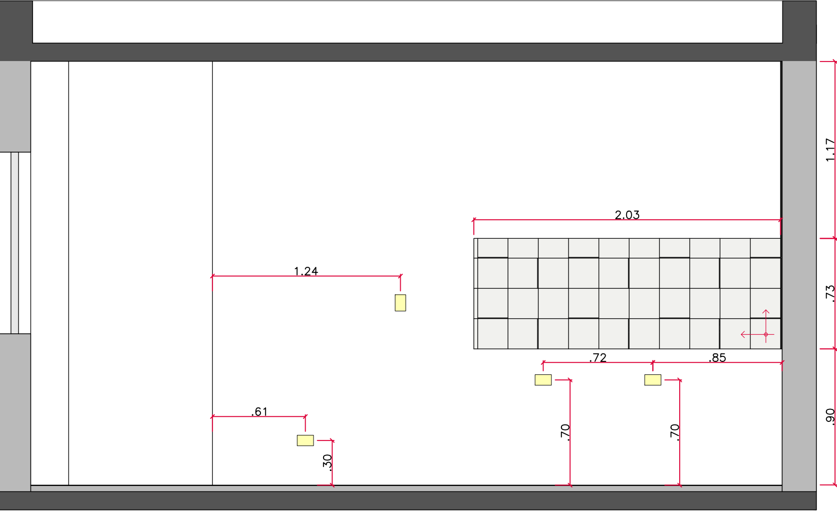
VISTA 02 - SERVIÇO esc 1:25
