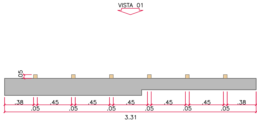
MA-18 PLANTA BAIXA esc 1:25
