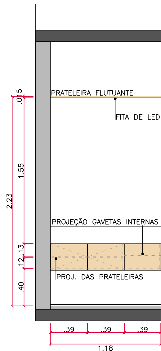
MA-13 E 14 VISTA 01 esc 1:25
