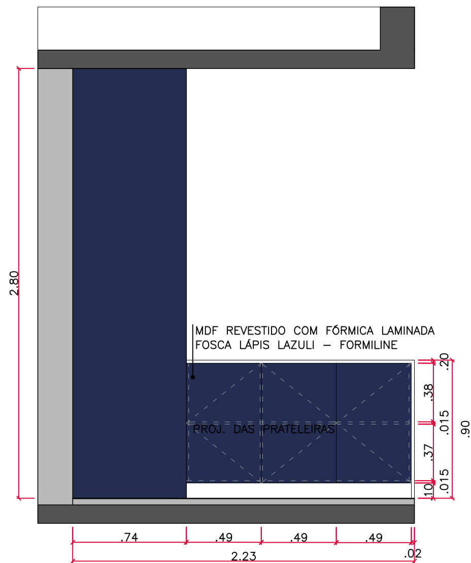
MA-01 VISTA 02 esc 1:25
