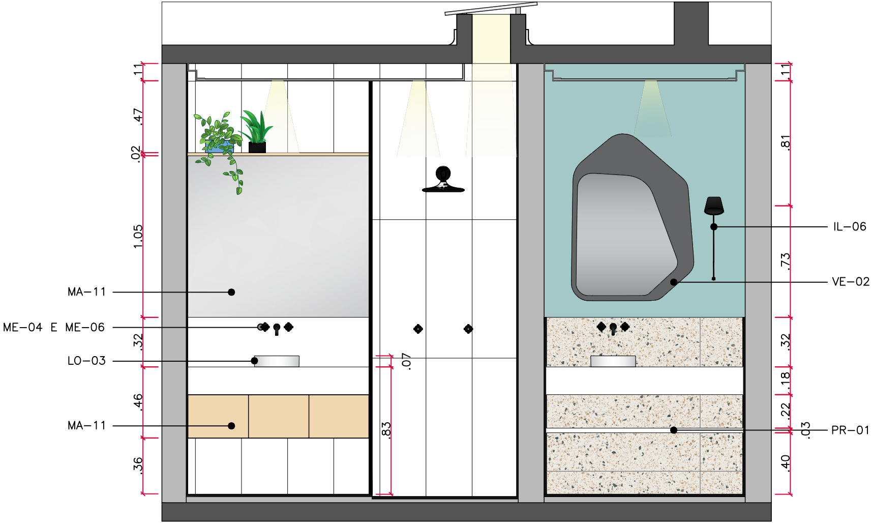
VISTA 01 - BANHEIRO esc 1:25
