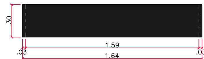
MA-10 VISTA 02 esc 1:20
