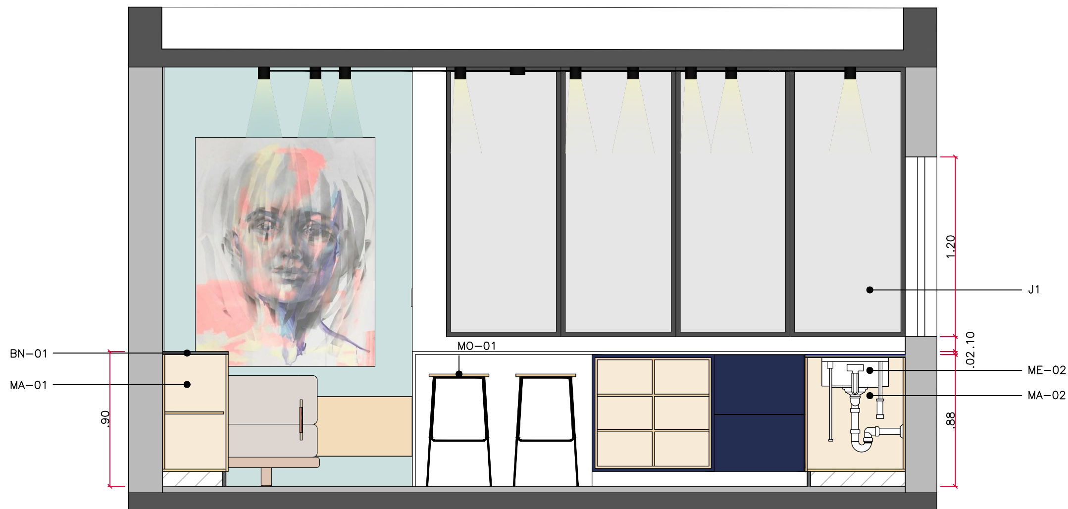
VISTA 01 - SERVIÇO esc 1:25
