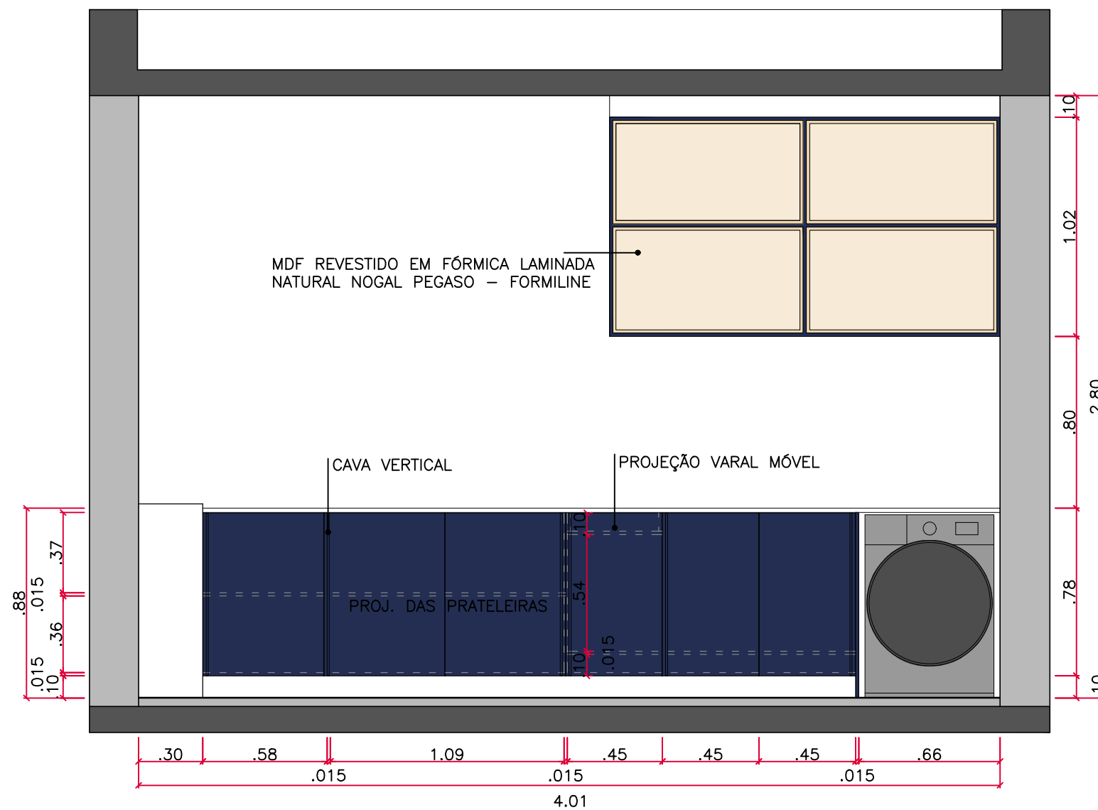
MA-02 E 03 VISTA 01 esc 1:25
